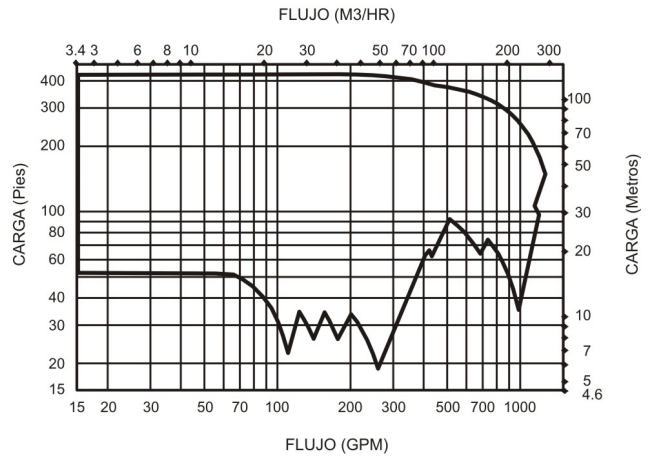
Gráfico de curvas Serie F - 3500 RPM
