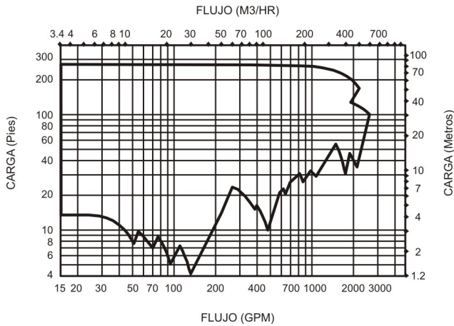
Gráfico de curvas Serie F - 1750 RPM
