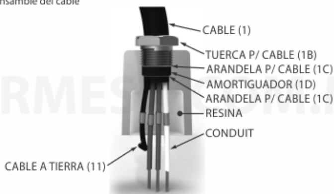
Figura 2: Ensamble del cable
