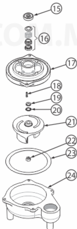
EXPLOSIONADO
