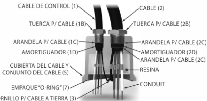
Figura 4: Cubierta de cable seccionada
