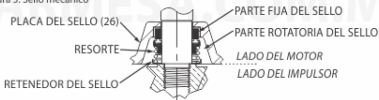
Figura 5: Sello mecánico
