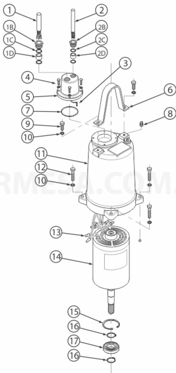
Figura 7: Dibujo explosionado.
