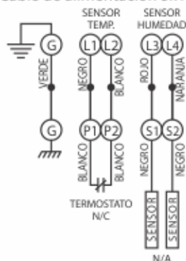
Cable de alimentación 5x18
