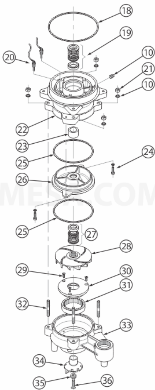
Figura 7: Dibujo explosionado (continuación).
