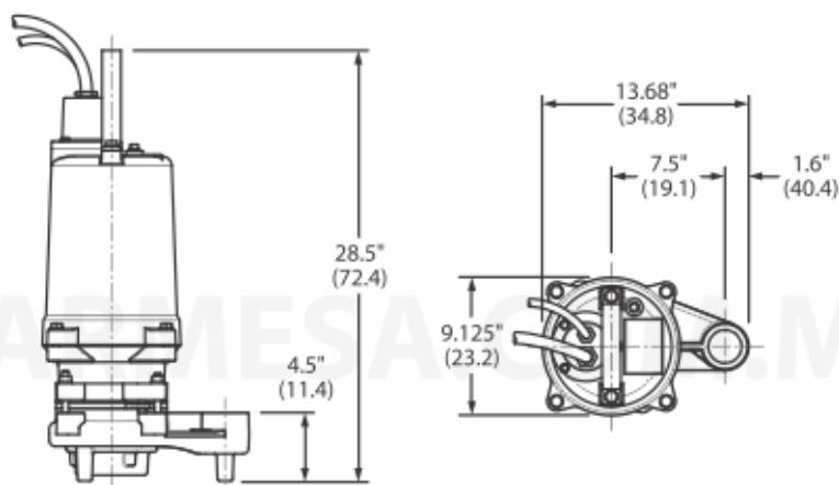
Figura 6: Dibujo dimensional.
